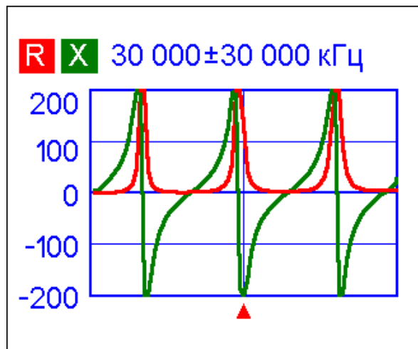
Короткозамкнутый кабель
